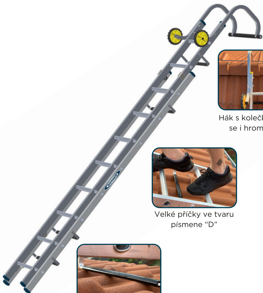
Pogumované opěrky, které oddálí žebřík o 8 cm od střešní krytiny
